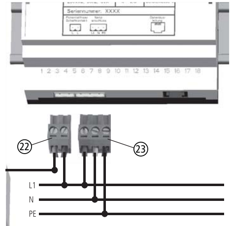
Abb. 5.4 Schalteinheit, elektrische Anschlüsse
