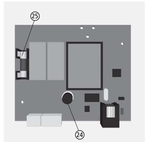
Abb. 5.5 Schalteinheit, elektrische Anschlüsse
