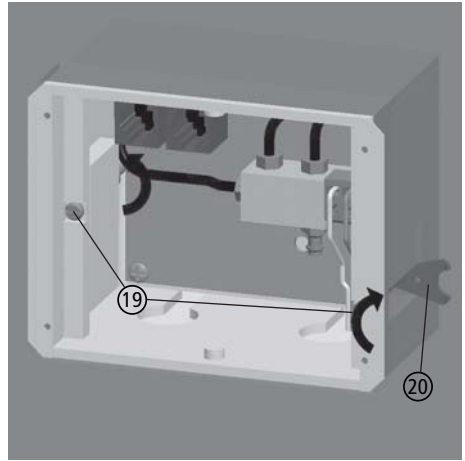
Abb. 4.8 Befestigungslaschen des Hohlwand-Gehäuses
